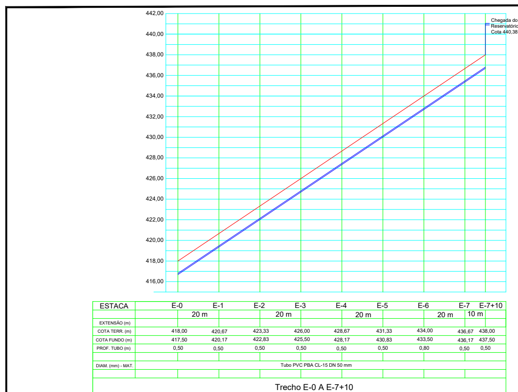
02 Perfil Longitudinal da Adutora ESCALA ..... 1/1
