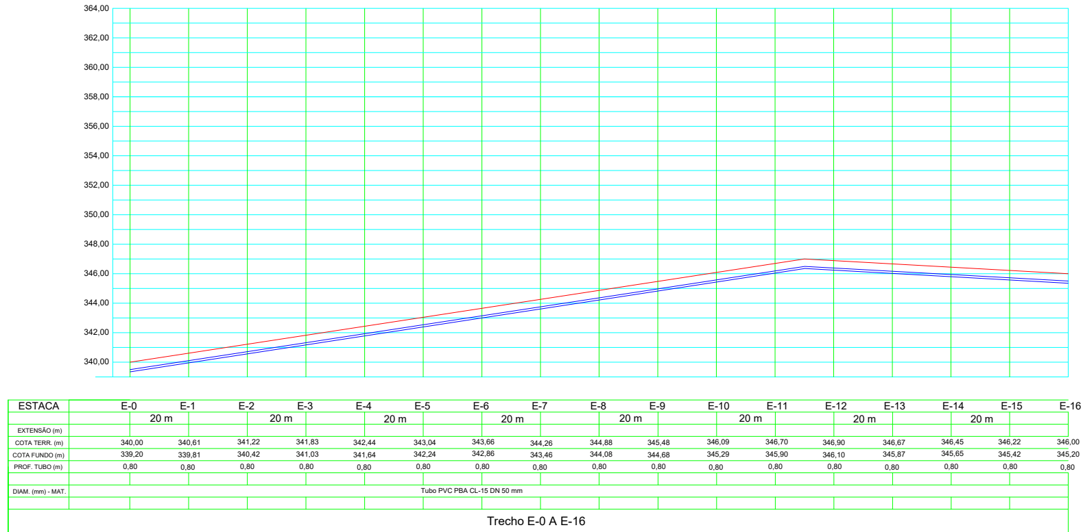
02 Perfil Longitudinal da Adutora ESCALA ..... 1/1
