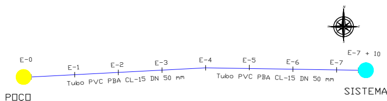
01 Planta Baixa da Adutora ESCALA ..... 1/1
