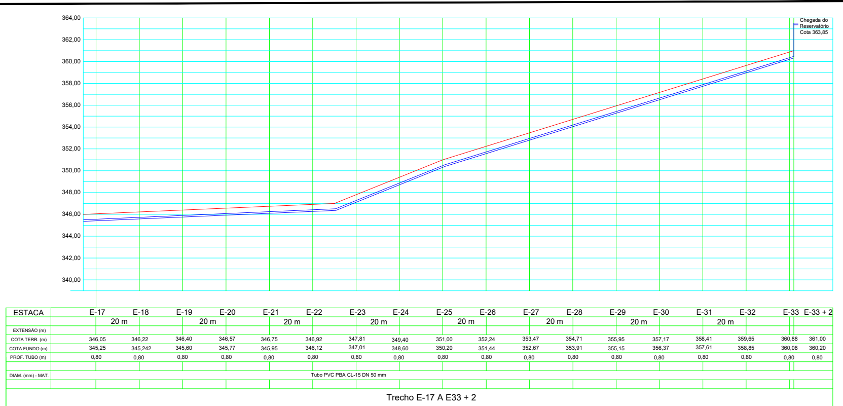
02 Perfil Longitudinal da Adutora ESCALA ..... 1/1
